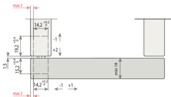
DOOR HEIGHT (mm)
