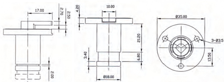
EG 104N กุญแจล็อกบานตู้ - ทับขอบ (FLAP LOCK)
