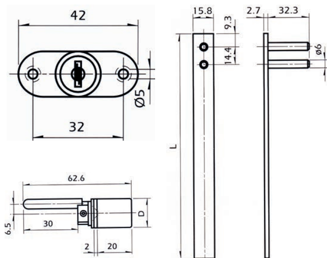
EG 110N กุญแจล็อกหน้า 3 ลื่นชัก FRONT CENTRAL LOCK
