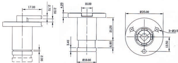
EG 104N กุญแจล็อกบานตู้ - ทับขอบ (FLAP LOCK)
