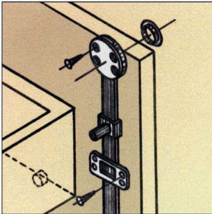
EG 109N กุญแจล็อกข้าง 3 ลื่นชัก SIDE CENTRAL LOCK
