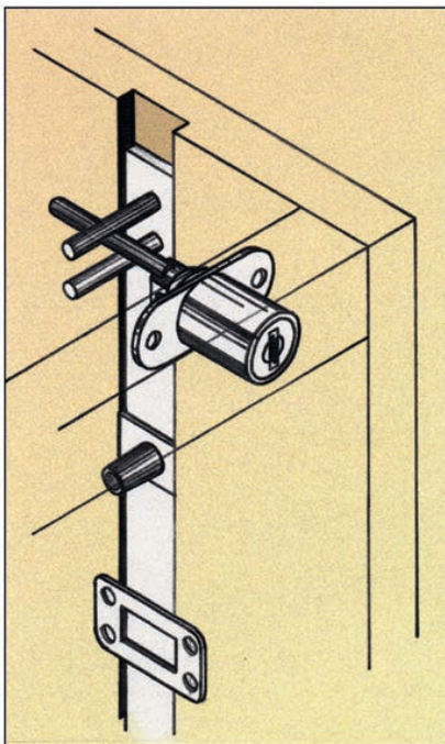
EG 110N กุญแจล็อกหน้า 3 ลื่นชัก FRONT CENTRAL LOCK
